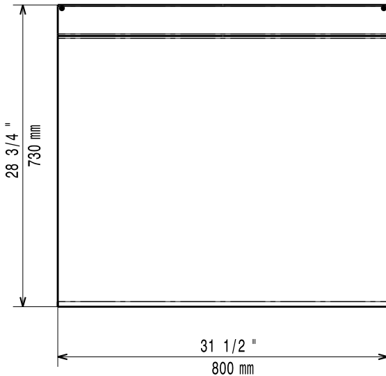
Felülnézet
