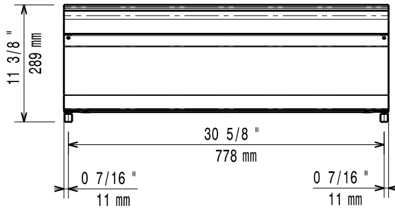
Oldalnézet
